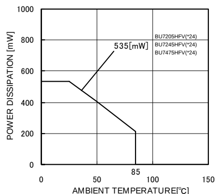
(d) BU7205HFV BU7245HFV BU7475HFV
