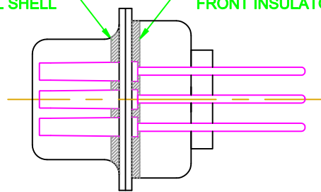
DETAIL A-A
