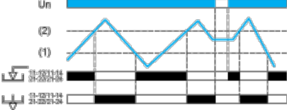
Fill/Empty function
