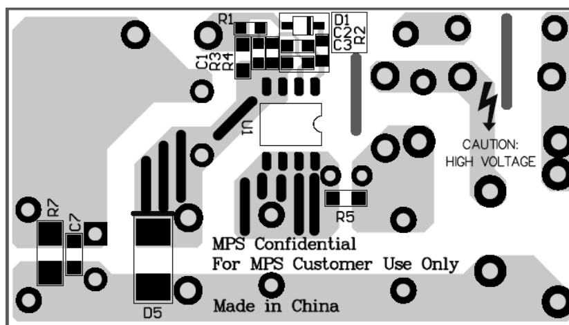
Figure 2 — Bottom Layer
