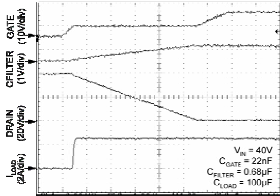
TIME (2.5ms/div.)
