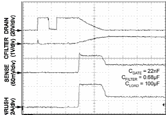
TIME (1ms/div.)
