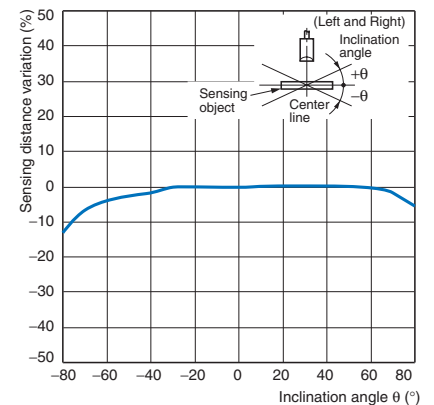
E3ZM-LS□4H(LS□9H)
