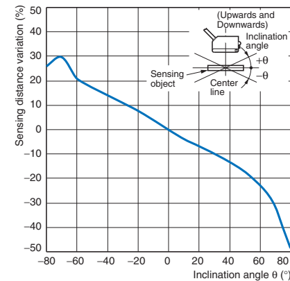
E3ZM-LS□2H(LS□7H)
