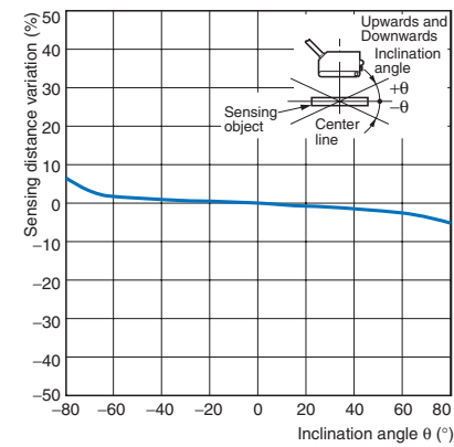
E3ZM-LS□1H(LS□6H)
