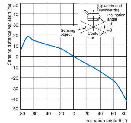
E3ZM-LS□4H(LS□9H)
