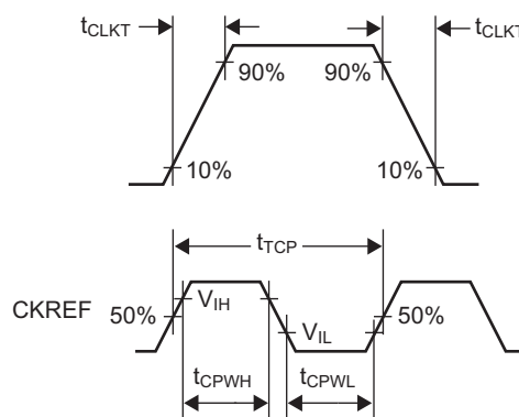
Figure 20. LVC MOS Clock Parameters
