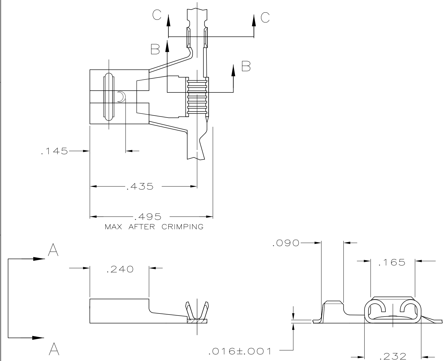
VIEW A-A
