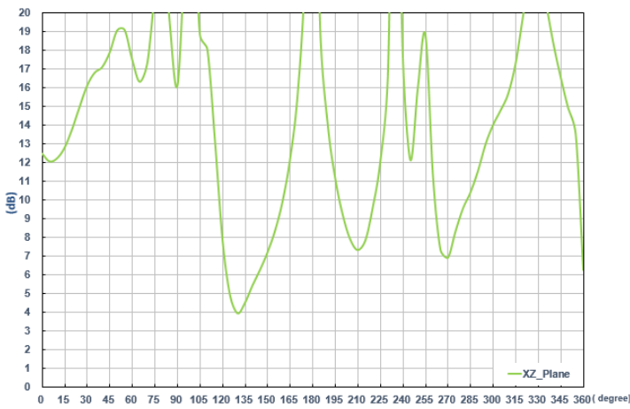
@1575MHz
