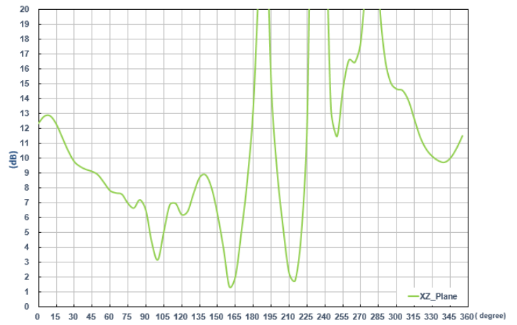
@1602MHz
