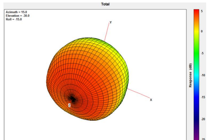
@1602MHz
