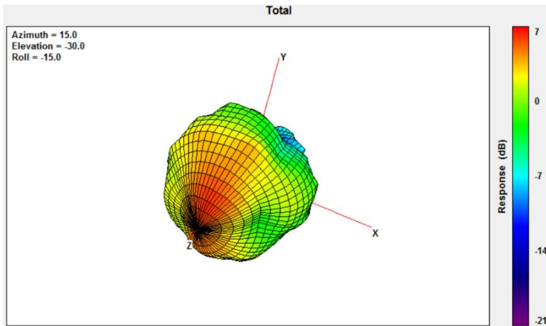
5550MHz
