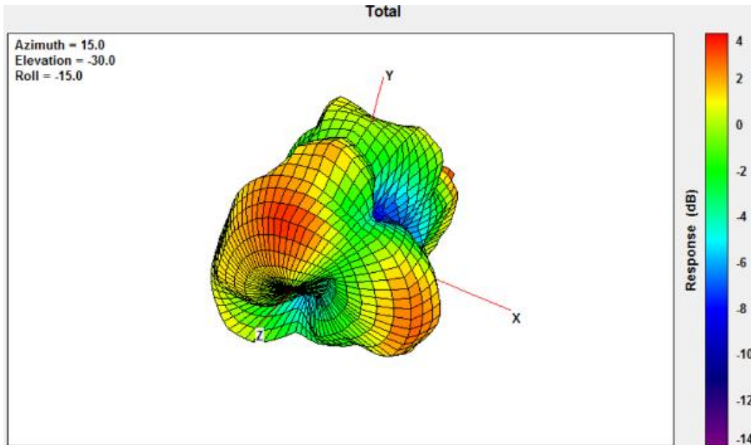
2450MHz
