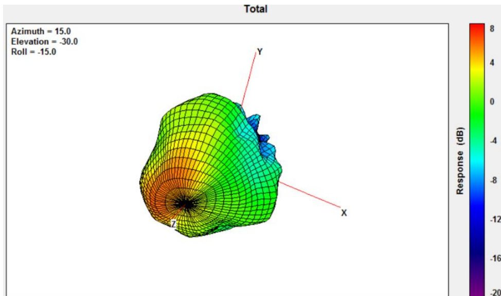
5550MHz
