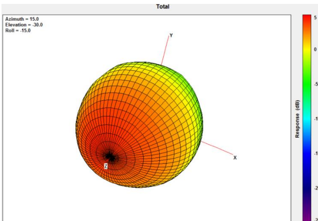
@1575MHz
