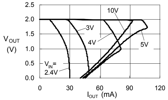
S-817A20A (Ta=25°C)
