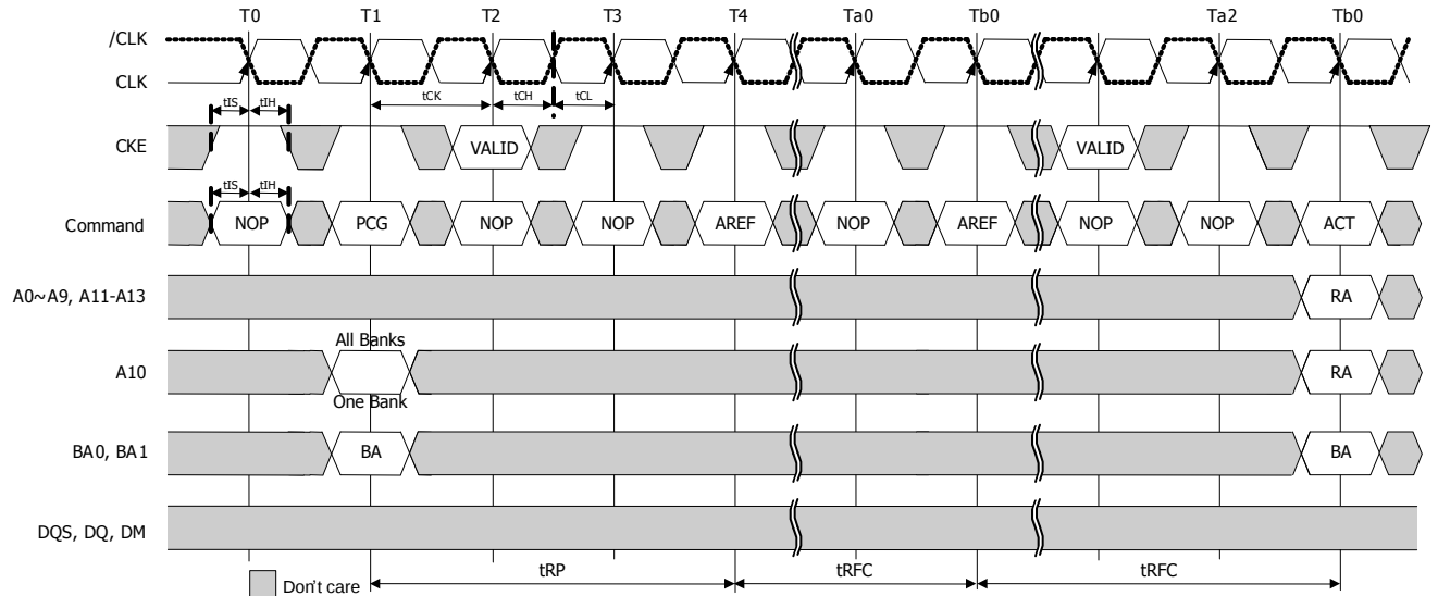
Figure33 : Auto refresh
