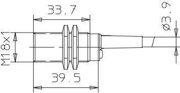
E2EL-X5□-L 2M, E2EL-X8□-DL 2M, E2EL-X8□-DSL 2M
