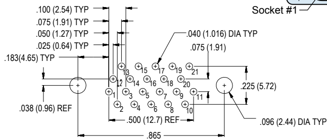
21 Socket M83513/31-C
