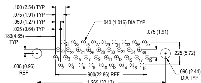
37 Socket M83513/31-F
