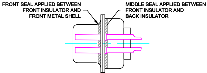
DETAIL A-A
