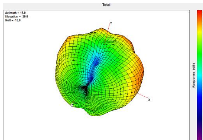
2500MHz
