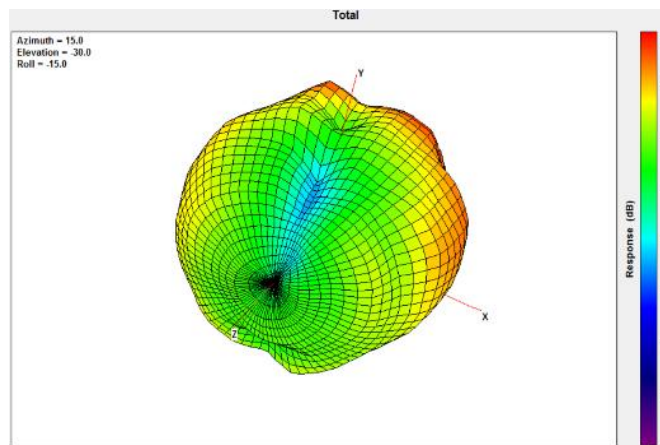
2450MHz
