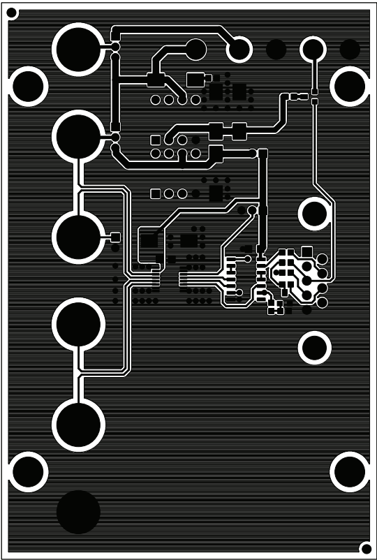
Top Layer
