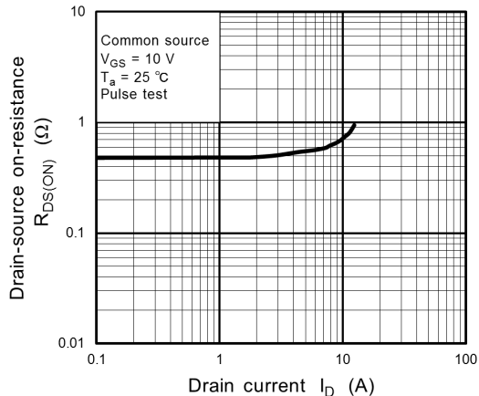
Fig. 8.6 R_{DS(ON)} - I_D
