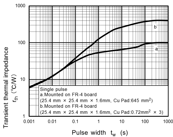
Fig. 7.11 r_{th} - t_w
