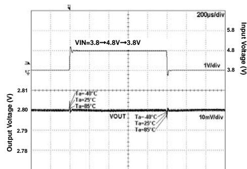
Fig 206. VIN Response
