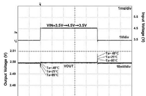
Fig 128. VIN Response
