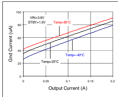
Fig 133. IOOUT - IGND
