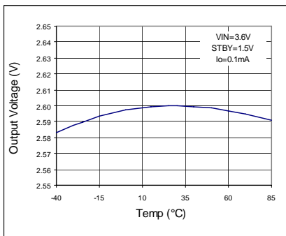
Fig 138. VOUT - Temp
