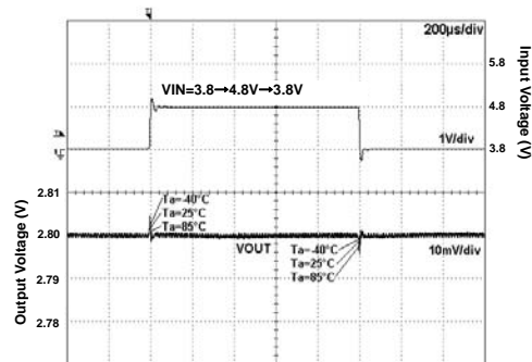
Fig 206. VIN Response
