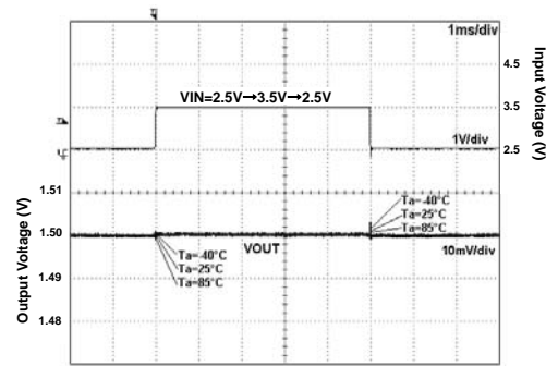
Fig 52. VIN Response
