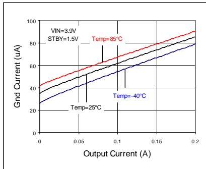
Fig 82. IOUT - IGDND
