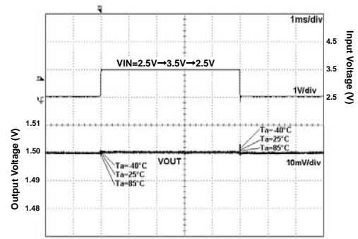
Fig 52. VIN Response
