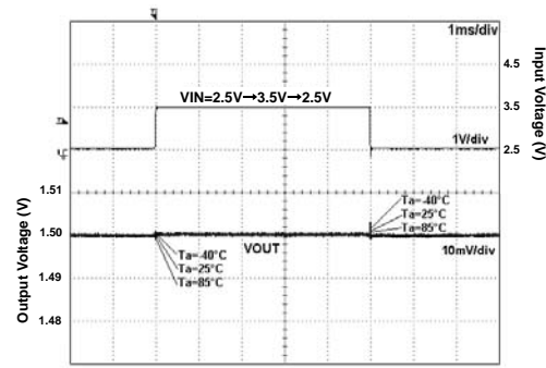
Fig 52. VIN Response
