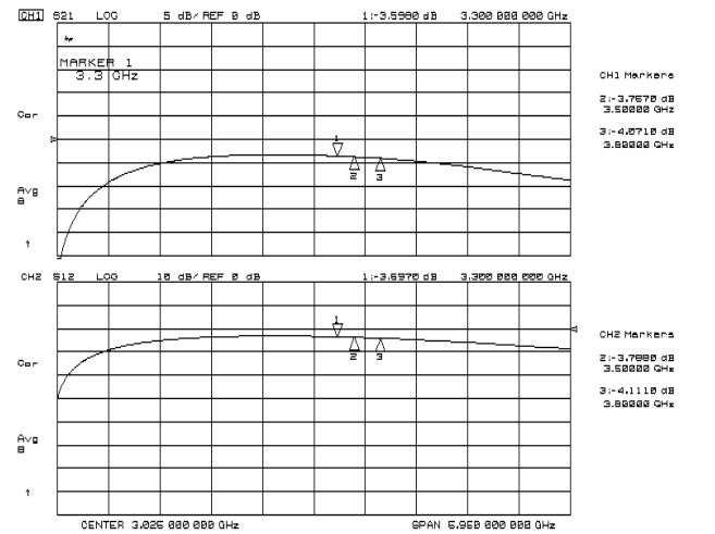
S21, S12
