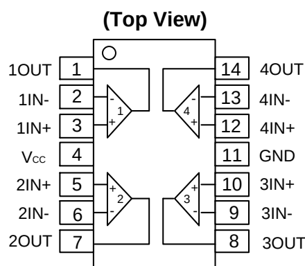
SO-14/TSSOP-14
