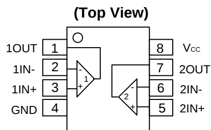
SO-8/TSSOP-8/MSOP-8
