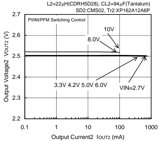
FOSC=300kHz, VOUT2=2.5V
