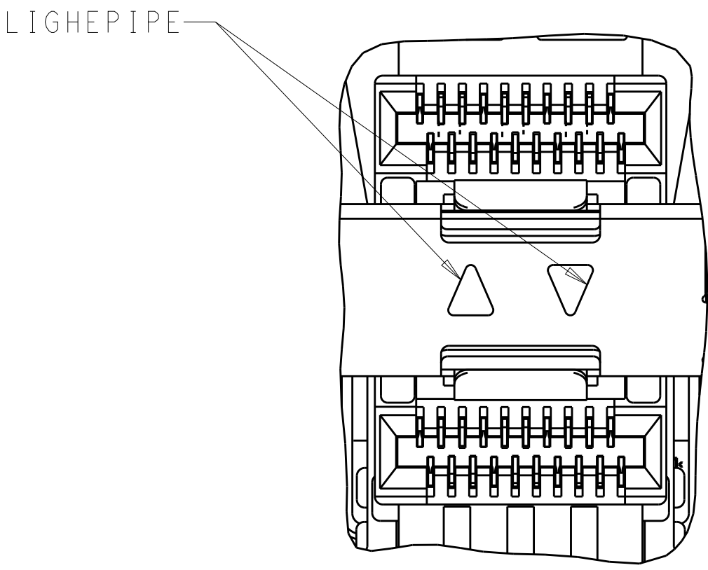
INNER LIGHT PIPES 2349202-3, 2349202-7 SCALE 5:1
