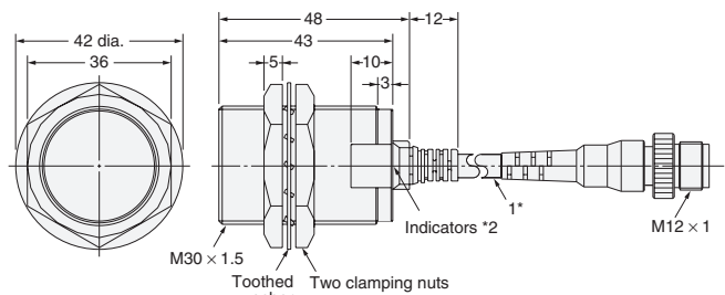
E2EQ-X15X1-M1(T)J
