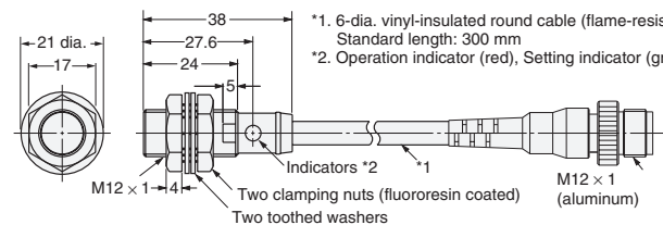
E2EQ-X10D1-M1(T)GJ
