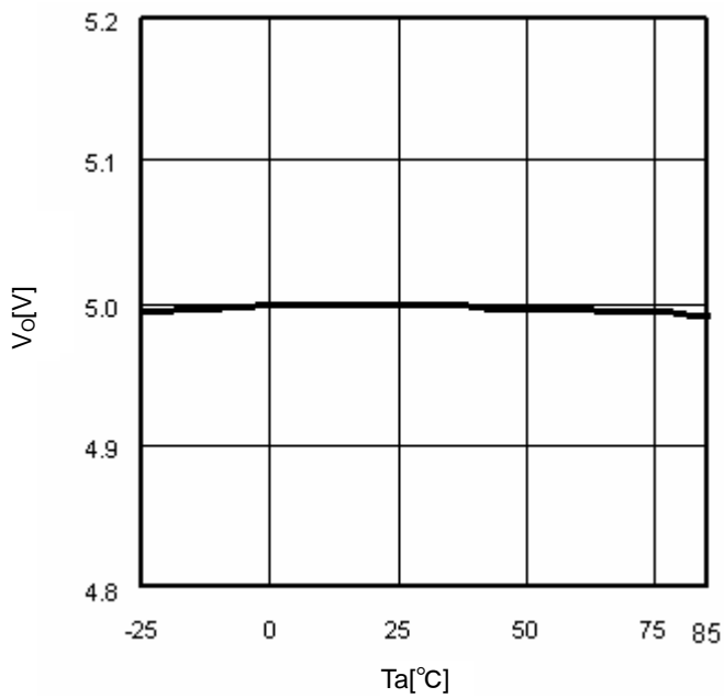
Fig.9 T_a-V_o ( I_o=0mA )
