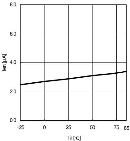
Fig.10 Ta-IEN
