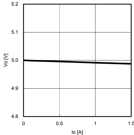
Fig.11 Io-Vo
