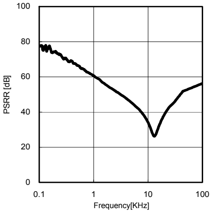
Fig. 19 PSRR (Io=0mA)
