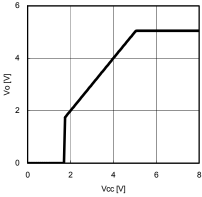
Fig. 13 Vcc-Vo (Io=0mA)
