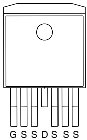
TO-263-7L
