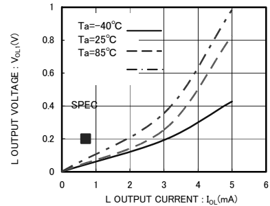
Fig.5 'L' output voltage V_{OL1} \sim OL_n ( V_{CC}=1.7V )
