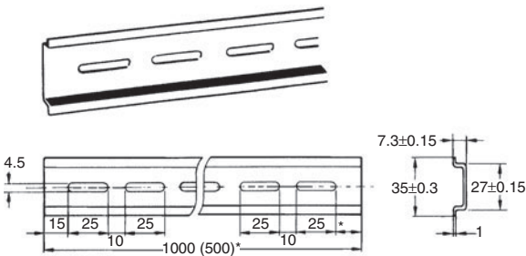
PFP-100N, PFP-50N (Conforming to EN 50022)
