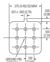
MGA/MGAD/MGADD HEADER
