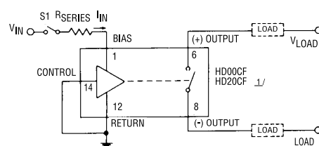
(D) 2 TERMINAL INPUT (DIRECT DRIVE)
