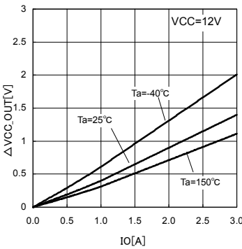
Fig.22 V(VCC-OUT)-Iout
