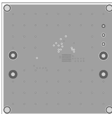
Figure 5—Bottom Layer
