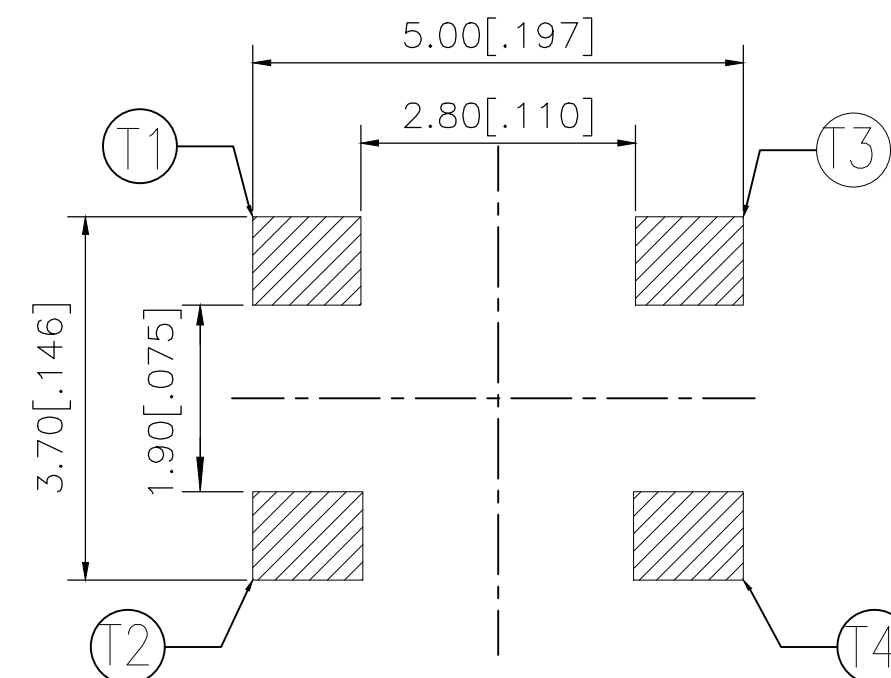
P.C.B. LAYOUT
