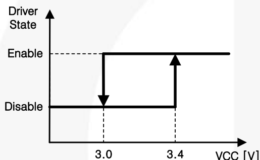
Figure 27. UVLO
