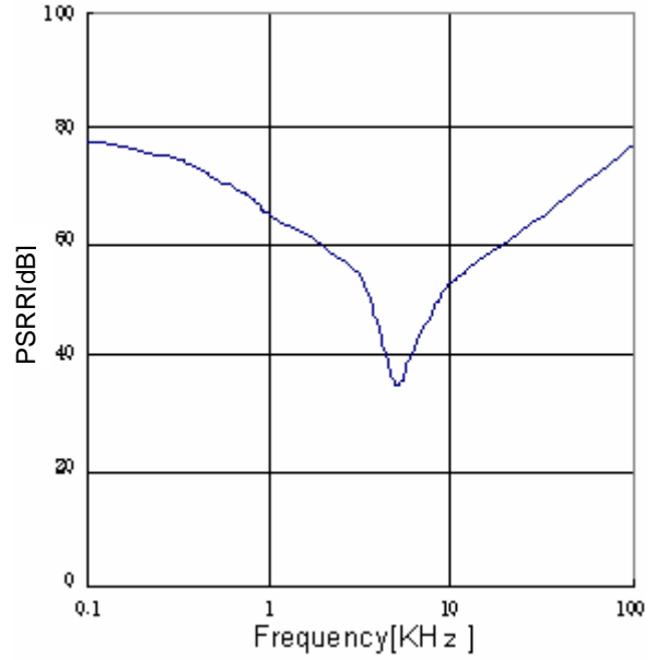
Fig.32 PSRR(Io=0mA)
