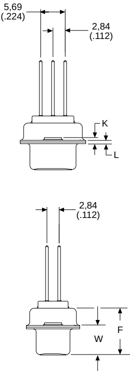
DD Configuration
