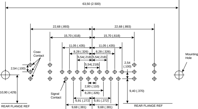
C 21WA4 17 #20 4 #8
