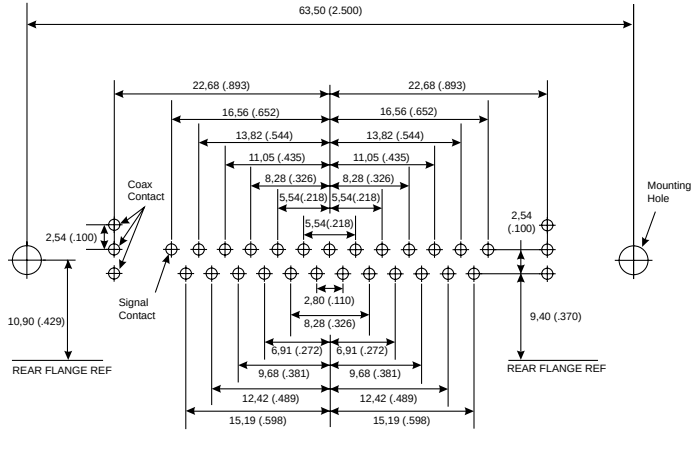
C 27W2 25 #20 2 #8
