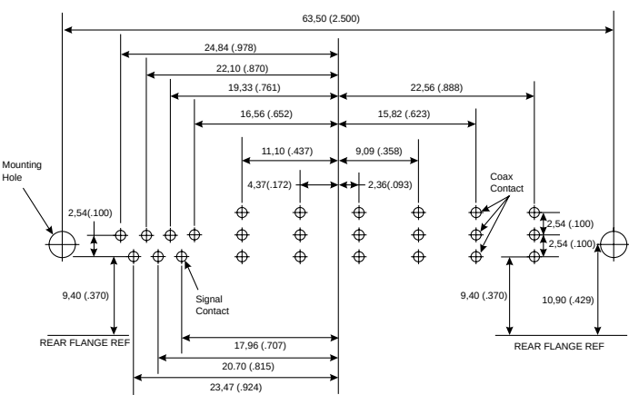
C 13W6 7 #20 6 #8
