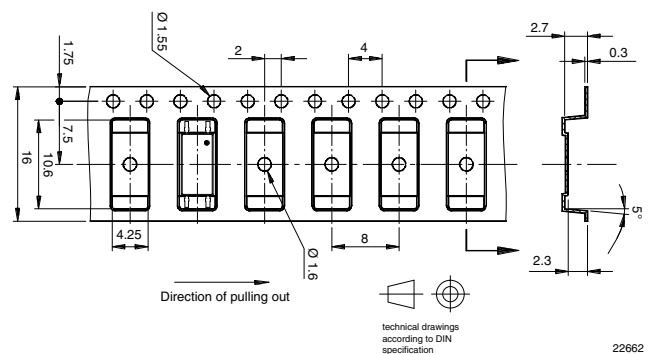
Fig. 21 - Tape Dimensions
